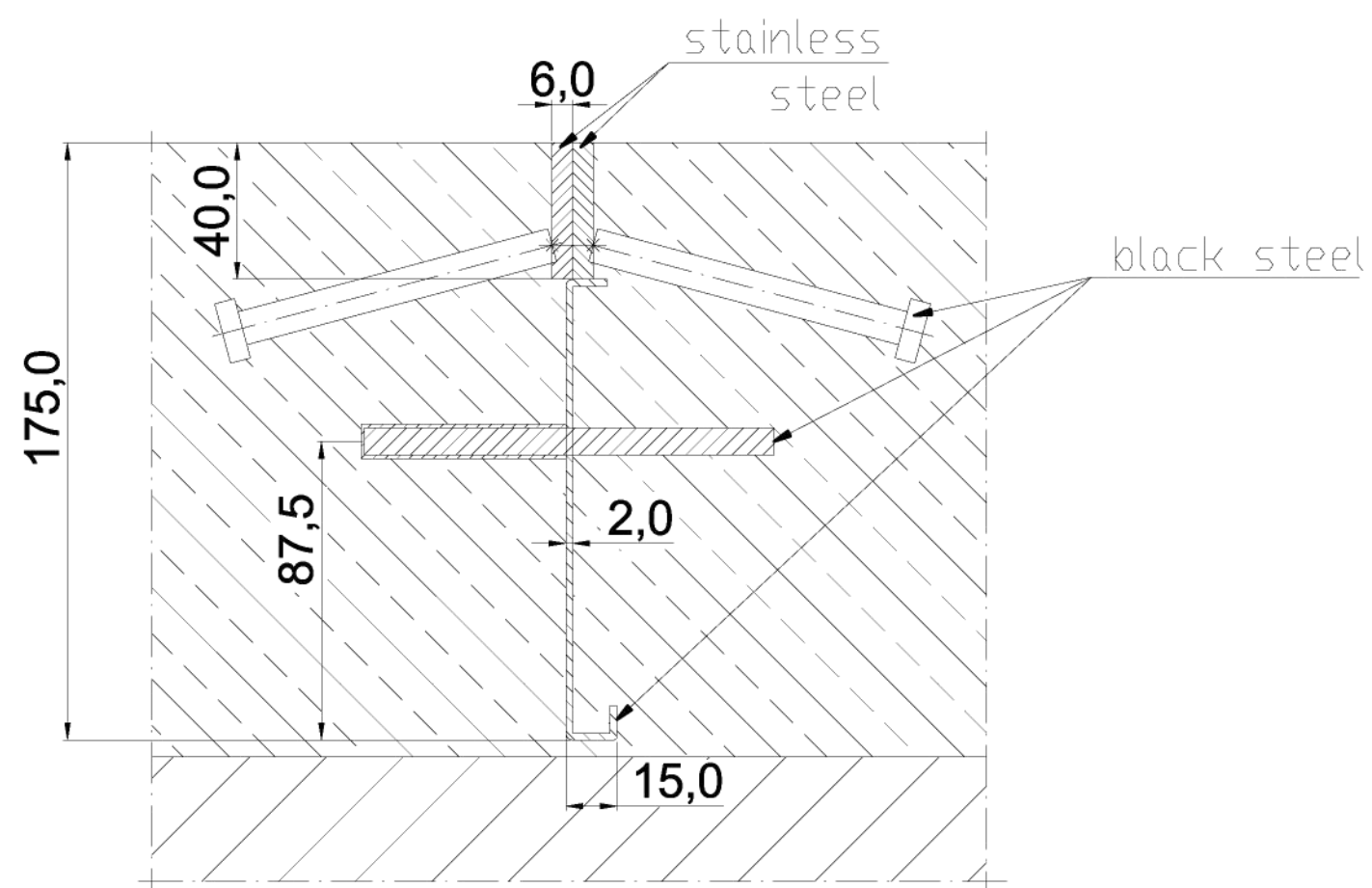
Conecto Dowel 06NA40-5D h=175 Section
